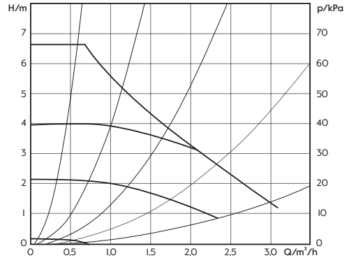
Характеристика циркуляційного насосу WIL0
