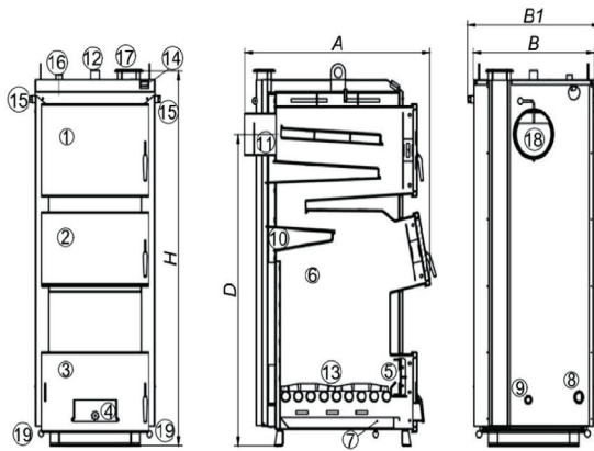
Рис.7 Vulcan VPSFW40 та його конструкція:
