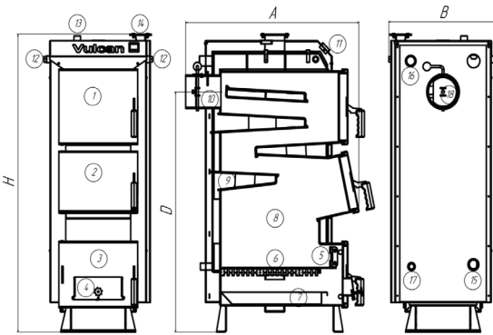
Рис.1 Vulcan SF15, SF18 та його конструкція:
