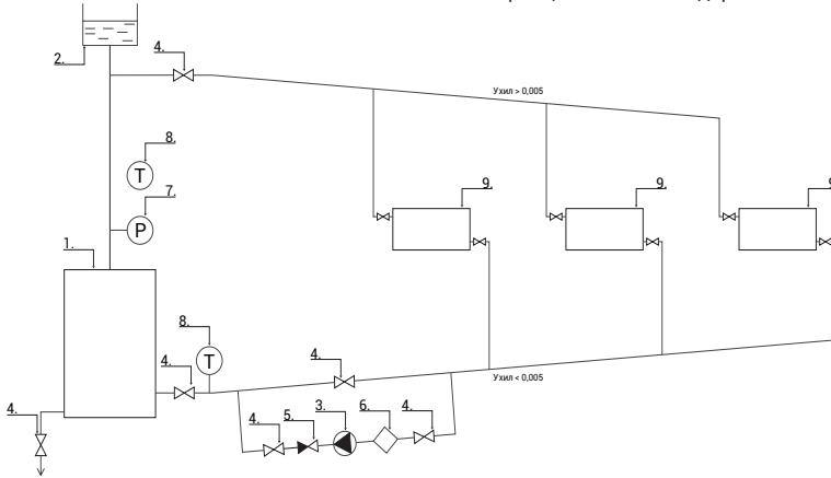
Рис.9 Принципова схема відкритої системи опалення
