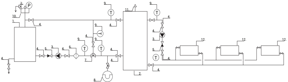
Рис.10 Принципова схема закритої системи опалення
