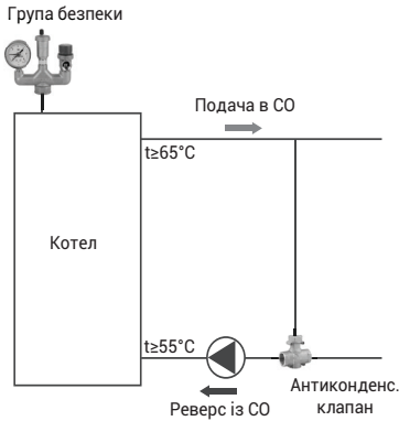
Рис.6 Схема з байпасом та антиконденсаційним клапаном
