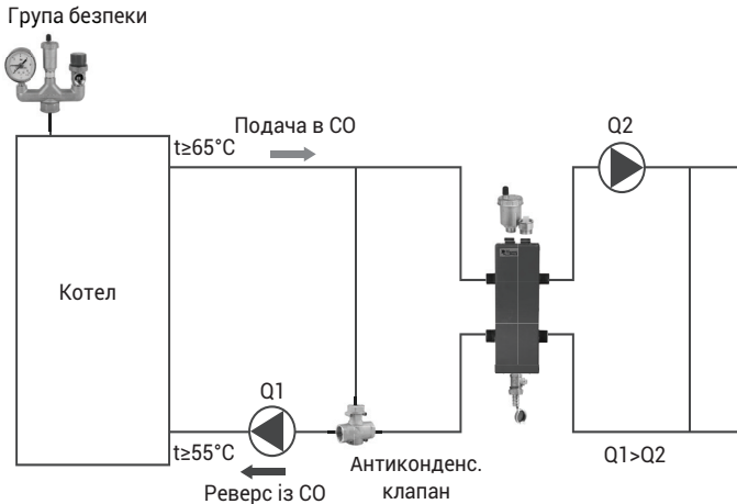
Рис.8 Схема з гідравлічним роздільником
