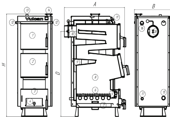
Рис.4 Vulcan VPSFW15, VPSFW18 та його конструкція:
