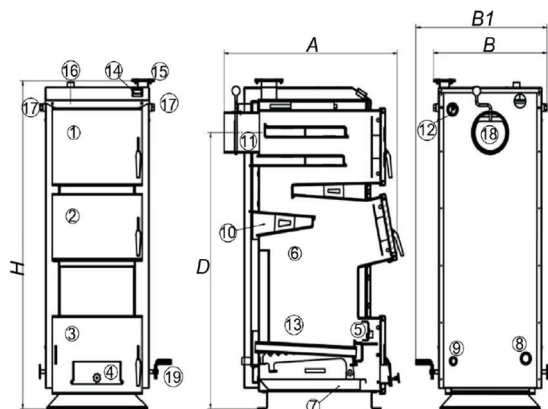
Рис.6 Vulcan VPSFW35 та його конструкція:
