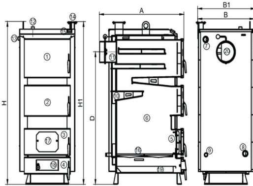
Рис.3 Vulcan SF40 та його конструкція:
