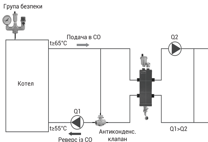
Рис. 4. Схема з гідравлічним роздільником
