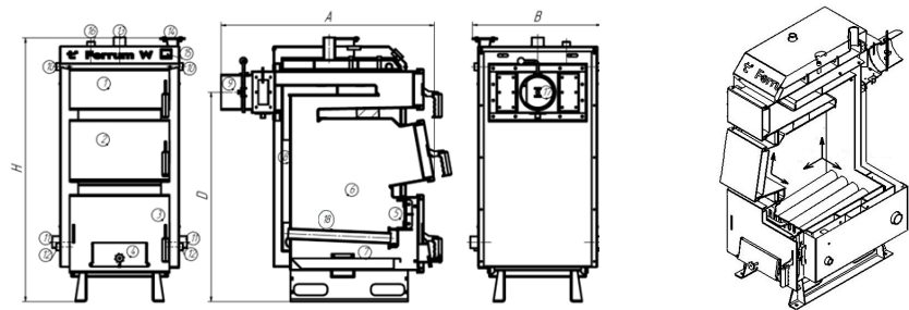
Рис.1 Ferrum W FW10, FW14, FW18, FW22, FW26, FW30 та його конструкція:
