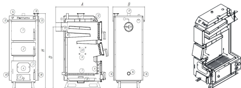
Рис.2 Ferrum+ FSF + 20, FSF + 26, FSF + 30, FSF + 35 та його конструкція:
