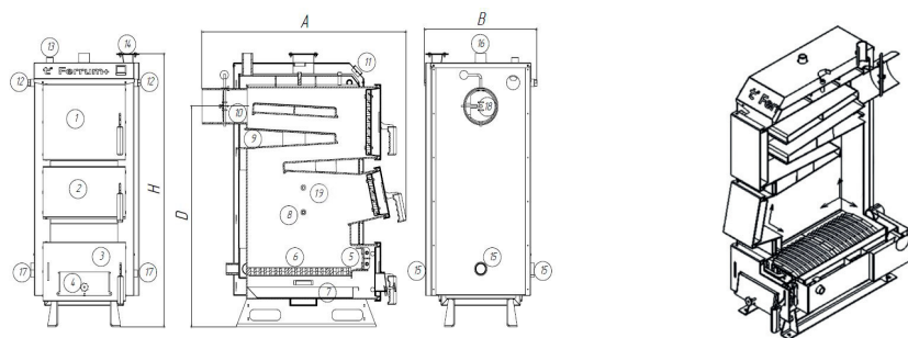
Рис.1 Ferrum+ FSF + 14, FSF + 16 та його конструкція:
