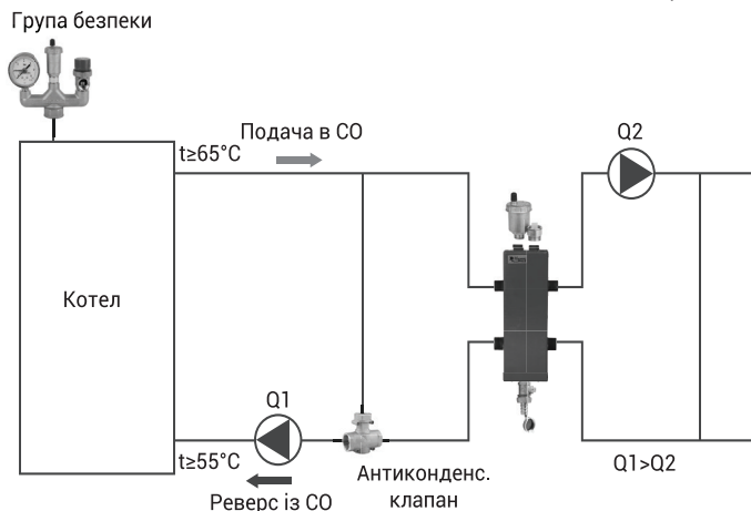
Рис.5 Схема з гідралічним роздільником
