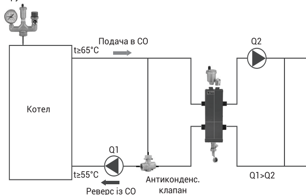
Рис.5 Схема з гідравлічним роздільником Група безпеки
