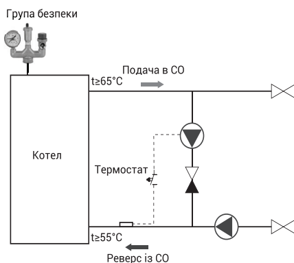
Рис.6 Підключення системи термічного розвантаження
