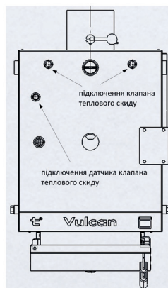
Рис.6 Підключення системи термічного розвантаження
