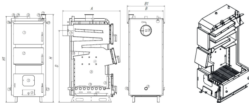
Vulcan VPSFW 50, VPSFW 40 та його конструкція:
