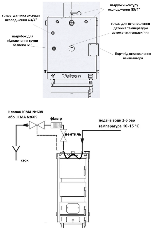
Рис.4 Патрубки для підключення та приблизна схема реалізації опції теплового розвантаження
