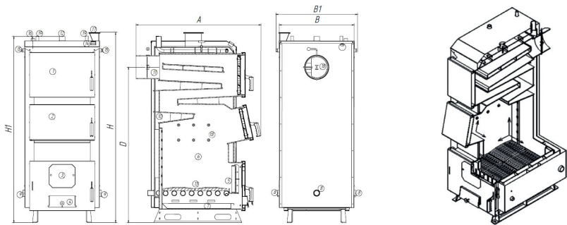
Vulcan VPSFW 60, VPSFW 70 та його конструкція:
